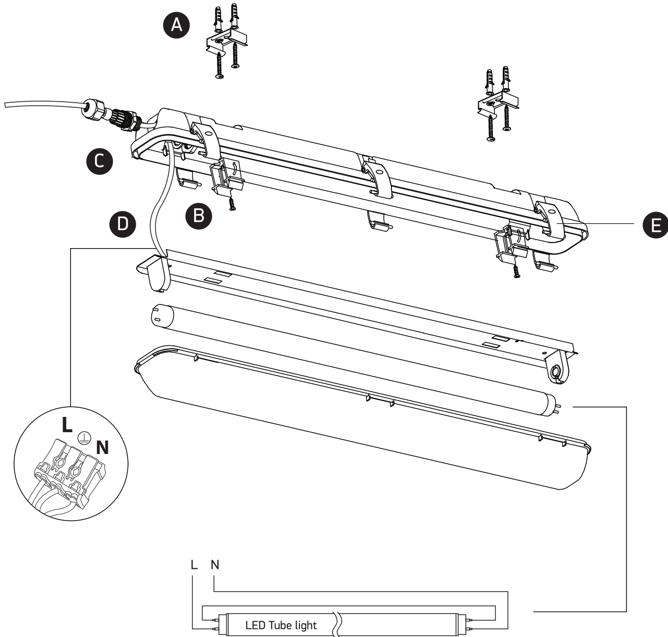
Wiring diagram.
