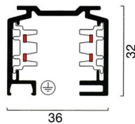
abmessungen_eutrac
