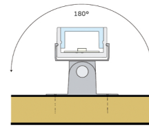
Montage mit schwenkbarer 180°-Halteklammer
