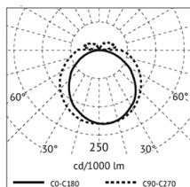
eckige Abdeckung
